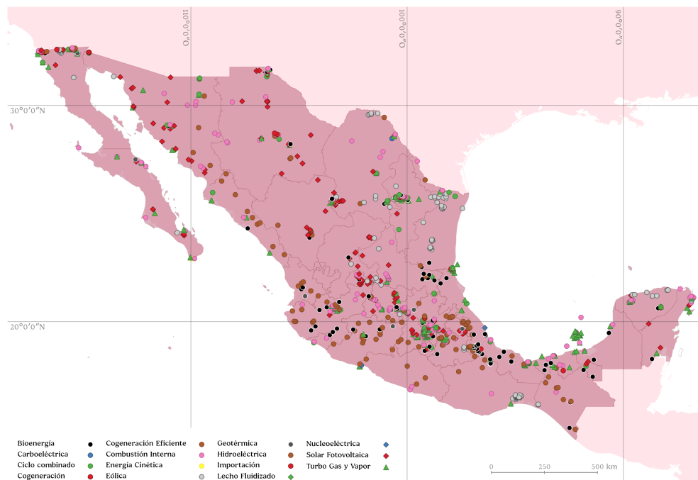
Figura 2.2 Centrales de generación eléctrica, 2024
